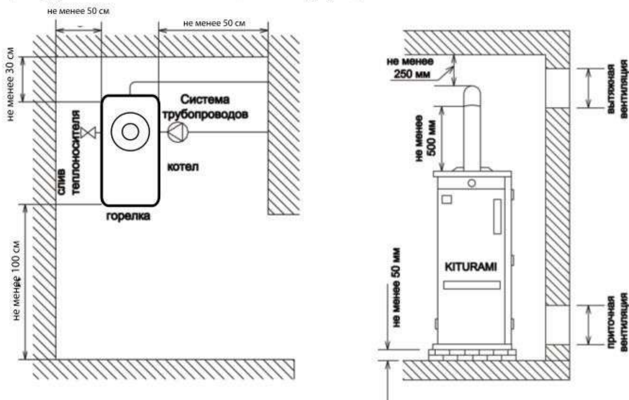
Рисунок 24. Установка котла
