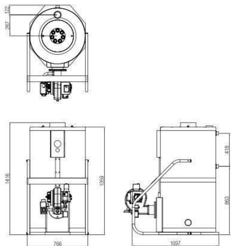
Рисунок 21. Габаритные и присоединительные размеры котлов KSG HIFIN-200
