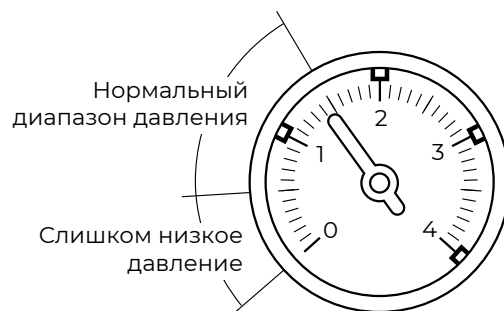
Рис. 8. Показания давления.
