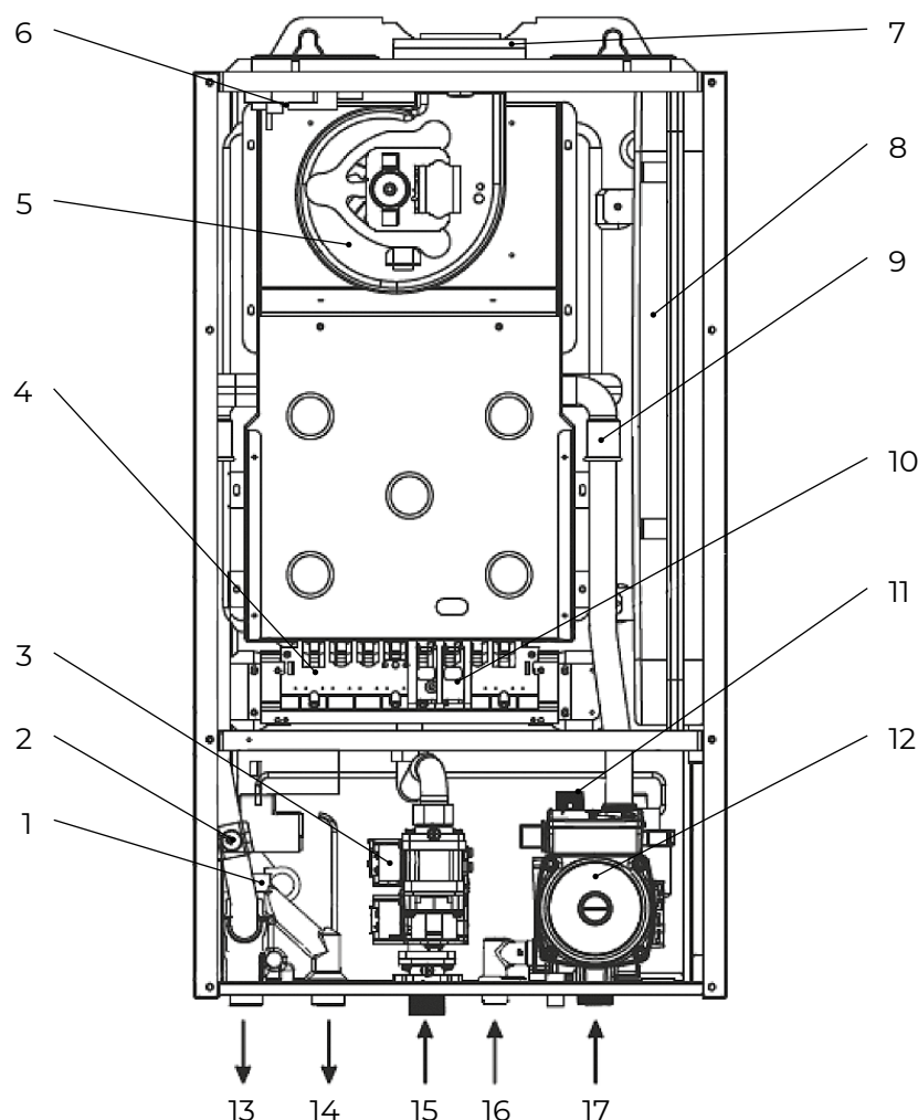
Рис. 4. Общая схема котлов B30 18 H, 24 H.
