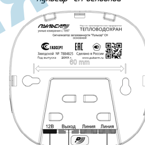
Сигнализатор загазованности «Пульсар» СН основной
