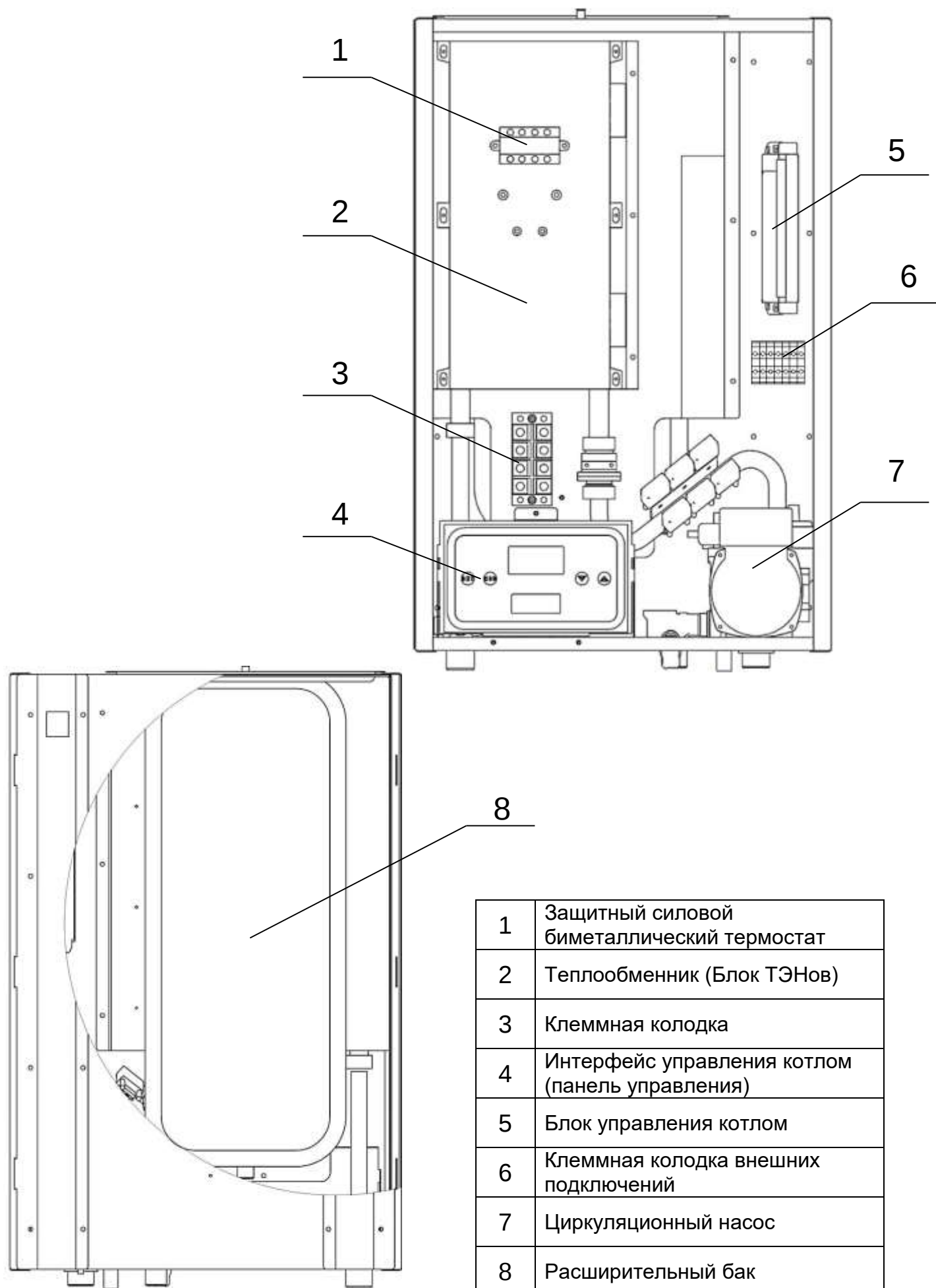
Рис. 2 Внутренне устройство
