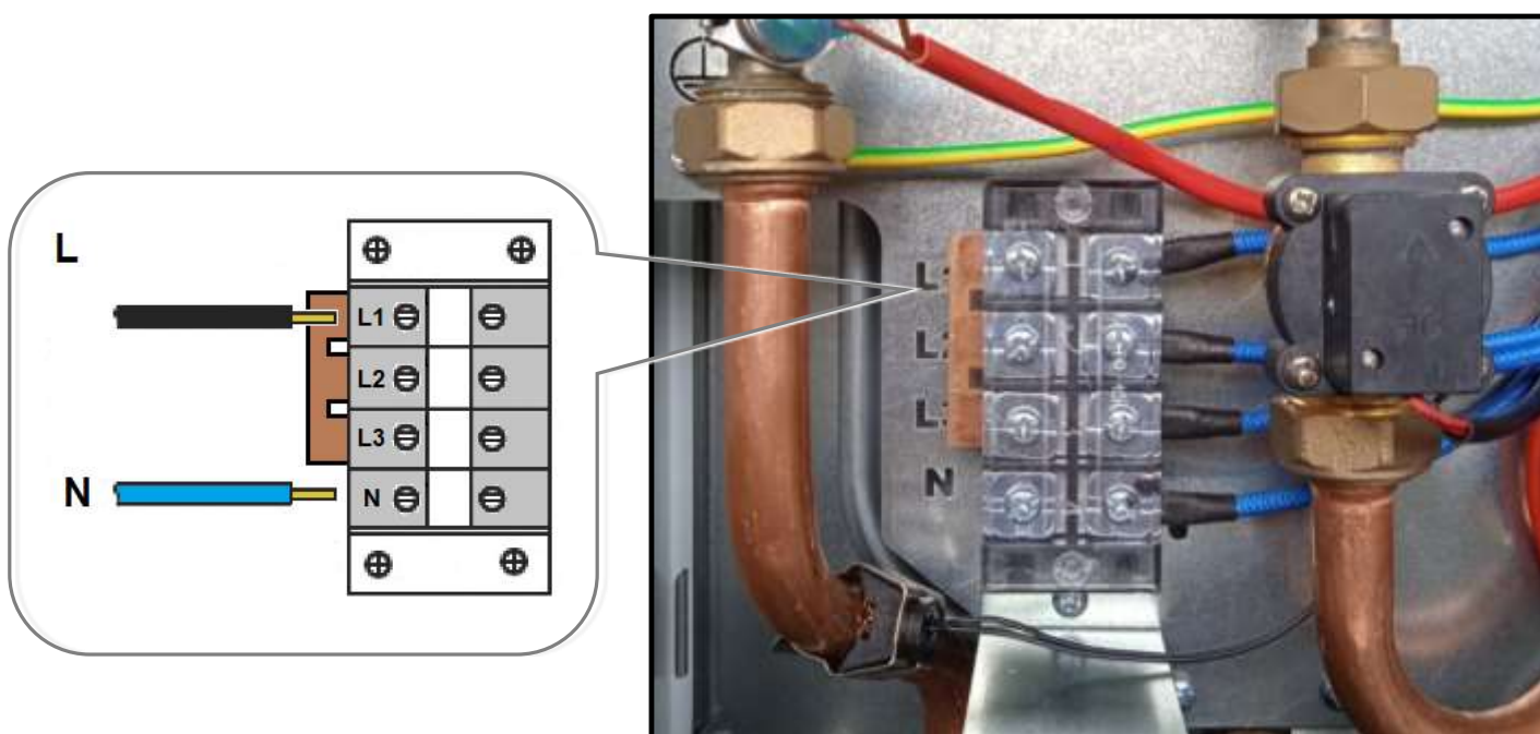
Рис. 15 Однофазное подключение
