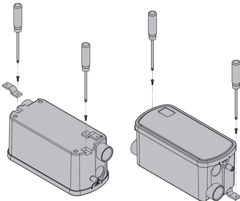
Рисунок 3 – Крепление КНС
