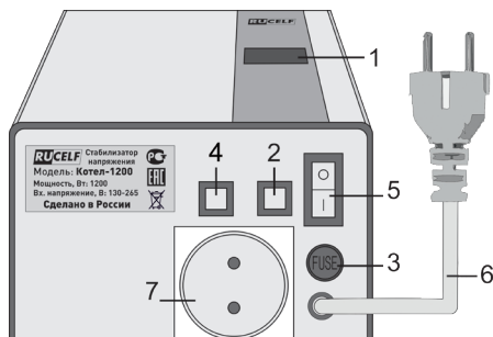
Рис. 1. Органы управления стабилизатора
