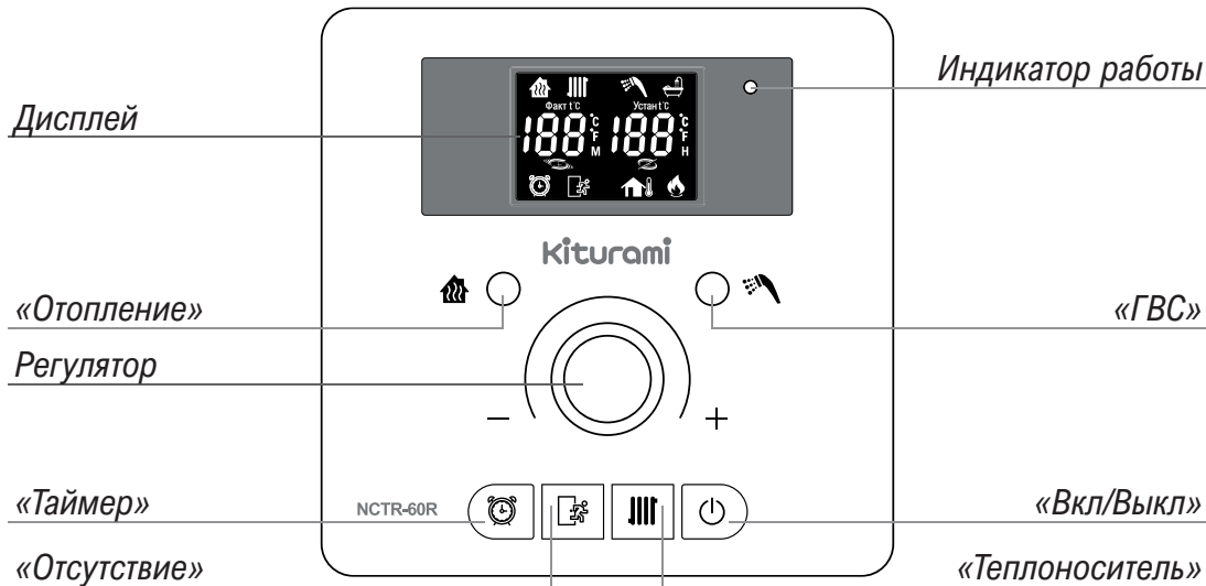
Рисунок 5. Пульт управления NCTR-60R.
