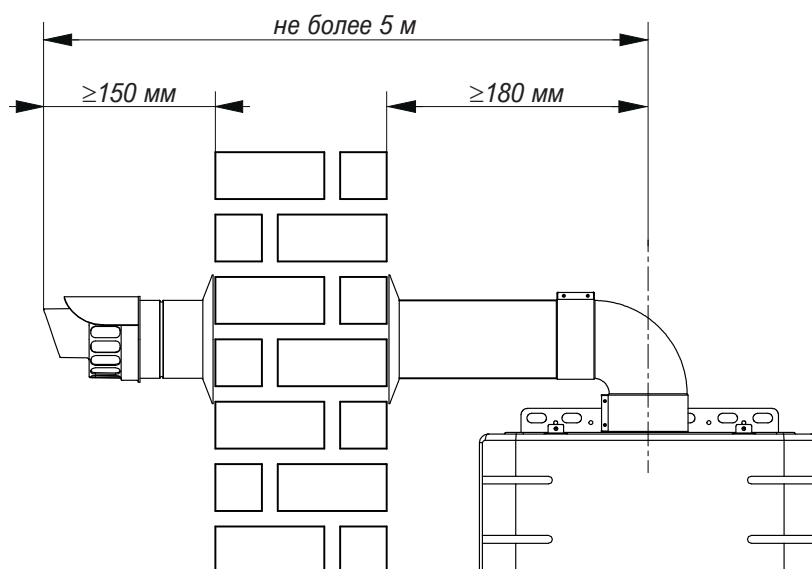
Рисунок 10. Коаксиальный дымоход.
