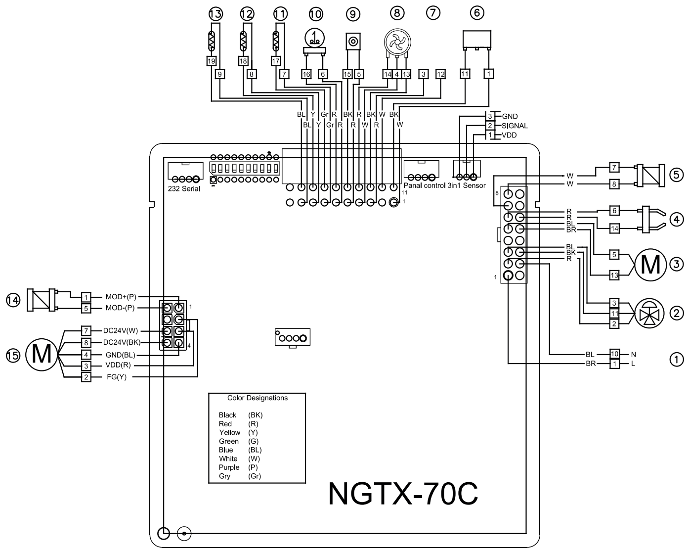
Рисунок 12. Схема электрическая.
